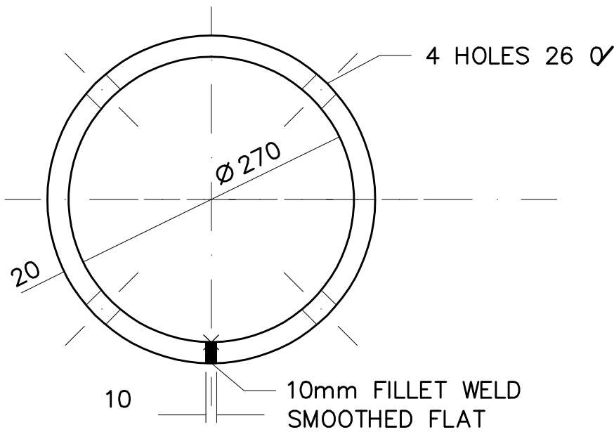
ELEVATION
